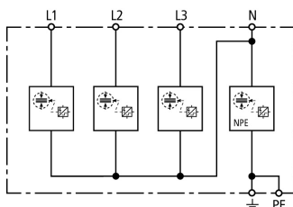
Esquema del DSH TT 255
