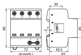
Dimensiones del DSH TT 255
