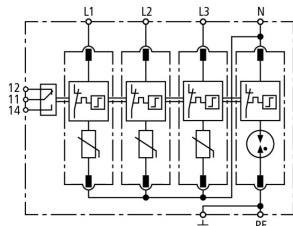
Esquema del DG M TT 275 FM
